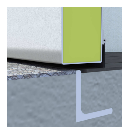
Przekrój: drzwi bezprogowe Kątownik 50/50/6mm ↓
