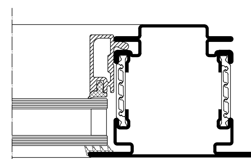
Przekrój pionowy F | vertical section F
