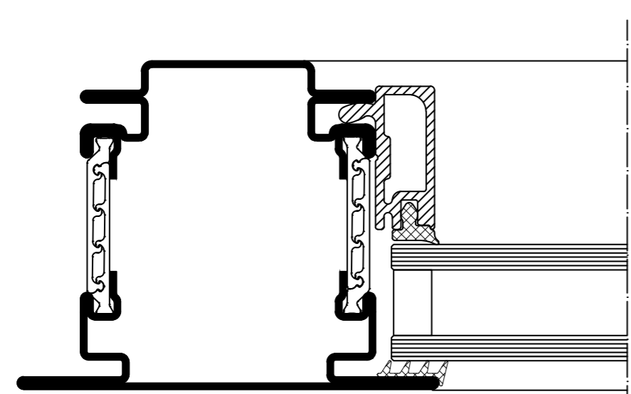
Przekrój pionowy D | vertical section D
