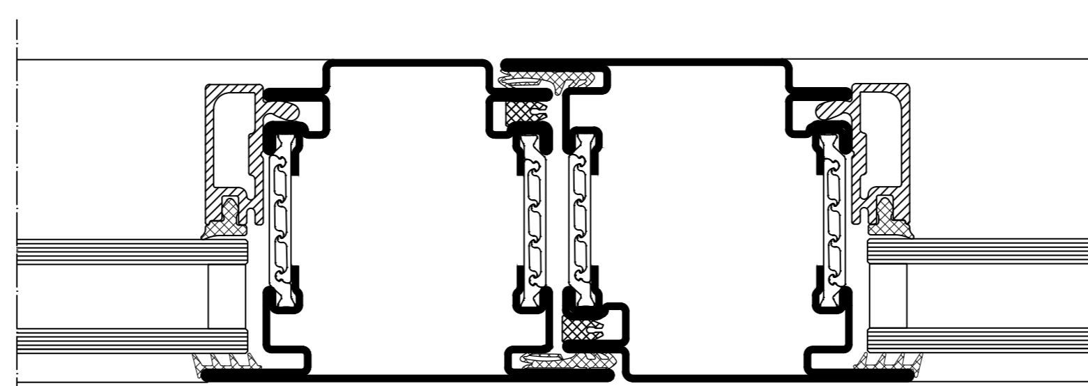
Przekrój pionowy E | vertical section E
