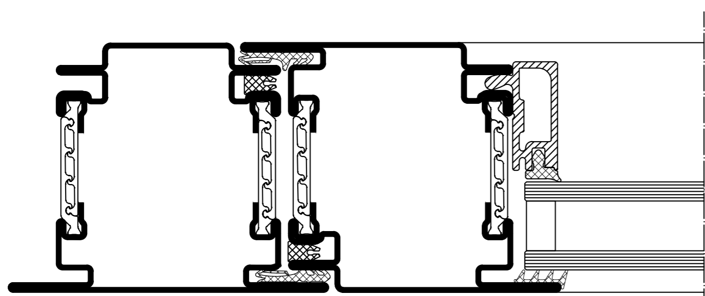
Przekrój pionowy B | vertical section B
